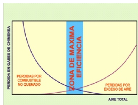
Figura 2: Zona de máxima eficiencia en la combustión
