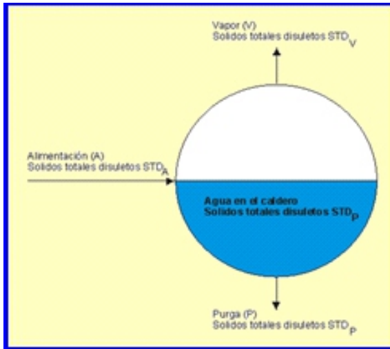
Figura 3: Recuperación del vapor Flash de las purgas
