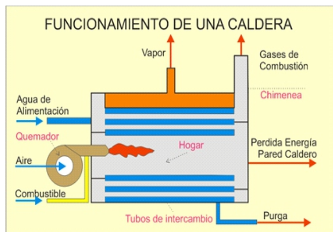
Figura 1: Corrientes de materia y energía en el Funcionamiento de una Caldera
