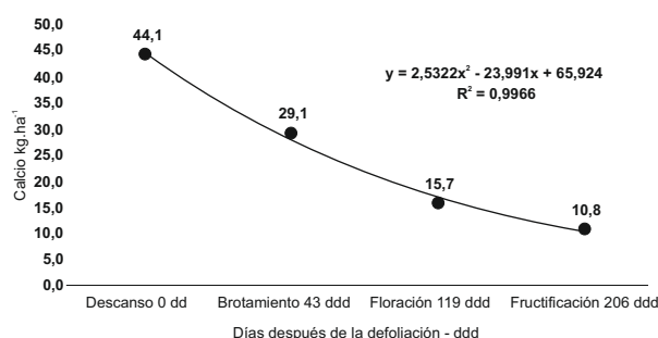
Figura 5. Absorción de calcio \text{kg.ha}^{-1} encada fase fenológica para camu camu.
