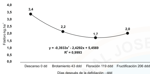
Figura 3. Absorción de fósforo \text{kg.ha}^{-1} encada fase fenológica para camu-camu.
