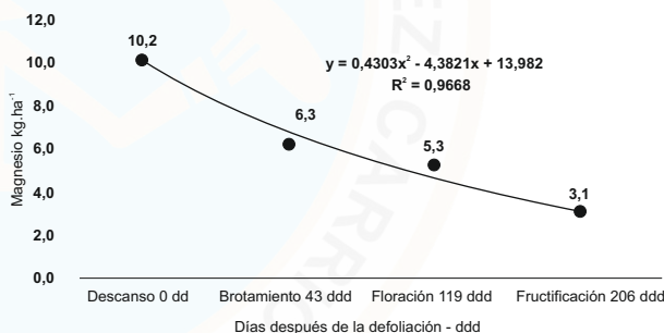
Figura 6. Absorción de magnesio \text{kg.ha}^{-1} en cada fase fenológica para camu camu.
